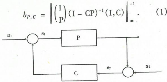
图 1 标准反馈结构
